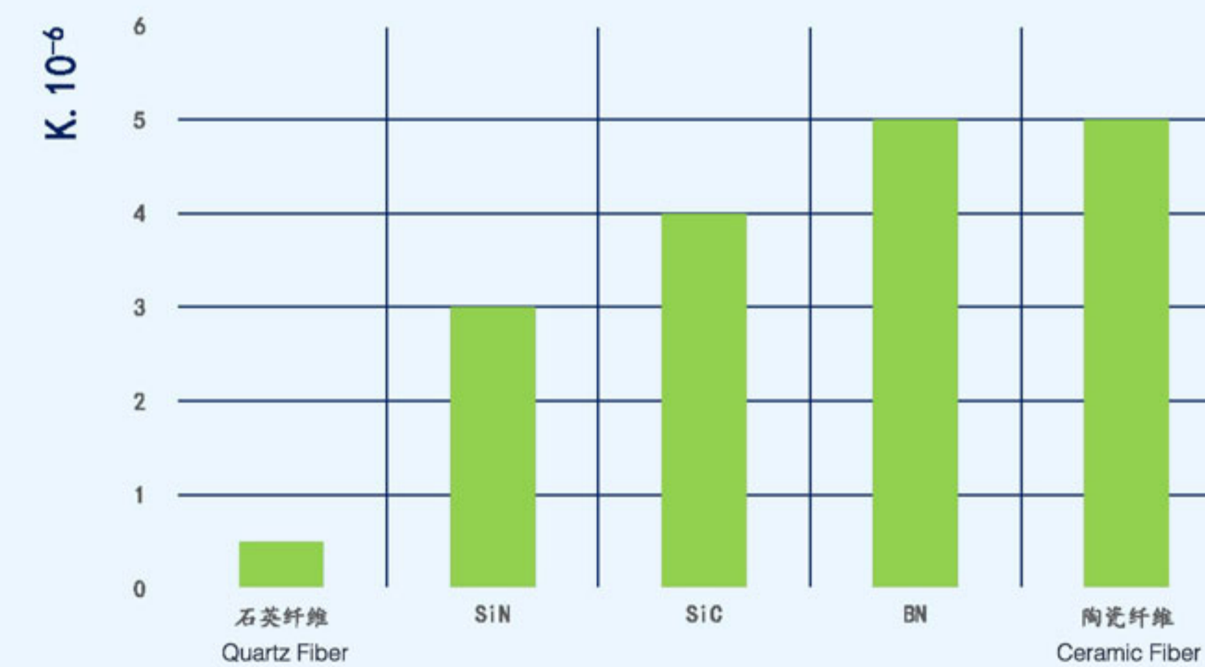
热膨胀系数 Thermal Expansion Coefficient
